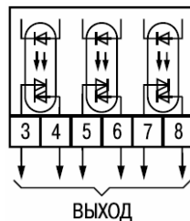
Рисунок Б.4 – Схема подключения ОВЕН TRM210-X.C3
